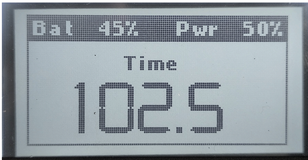
Figura 3.2 — Display LCD del LucchiMeter BASIC durante una misurazione, con indicazioni di Bat, Pwr e tempo Time in microsecondi
